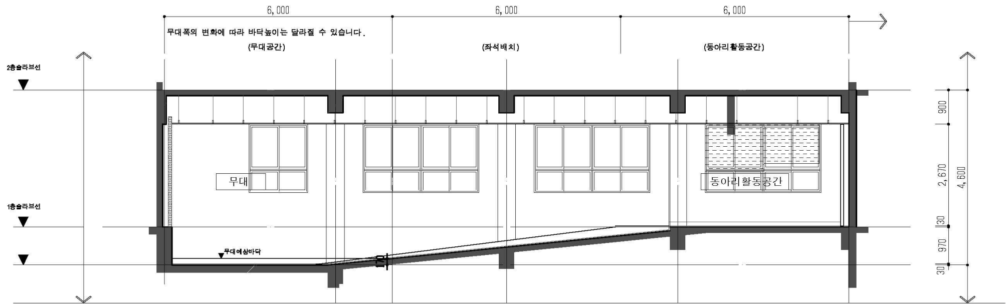
기존시청각실 단면
